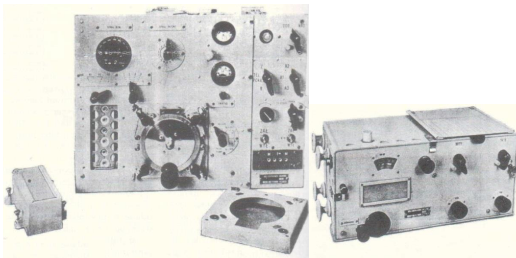
Radiostacja NI L/L (z prawej – nadajnik, z lewej – odbiornik)
