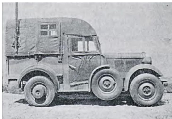
Radiostacja N2/S
